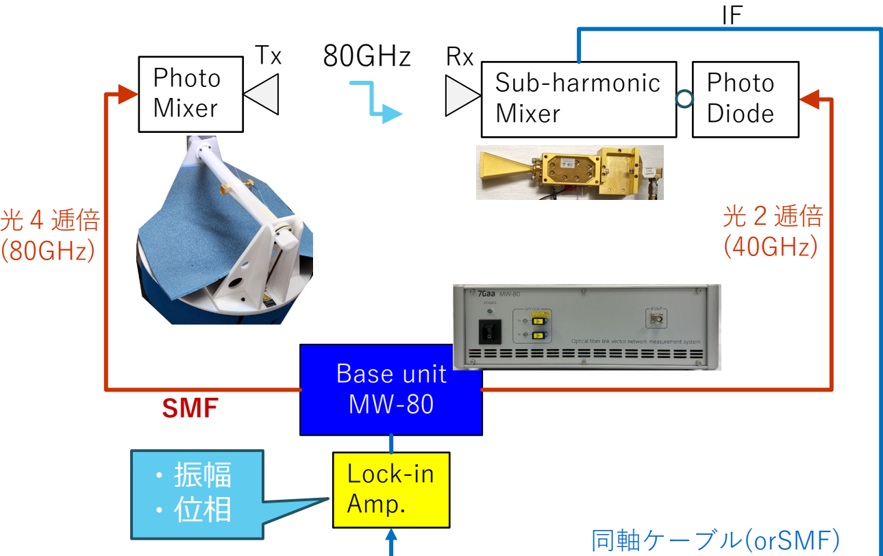
システム構成例(80GHz帯)
